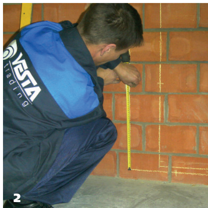
2 В соответствии с проектом намечаются места установки неподвижных и подвижных опор
